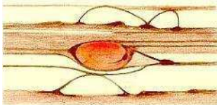
TMO/JPL/NASA
