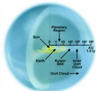
Oort Cloud
