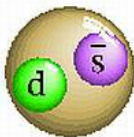
K^0
