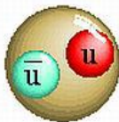
\pi^0
