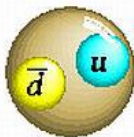
\pi^+
