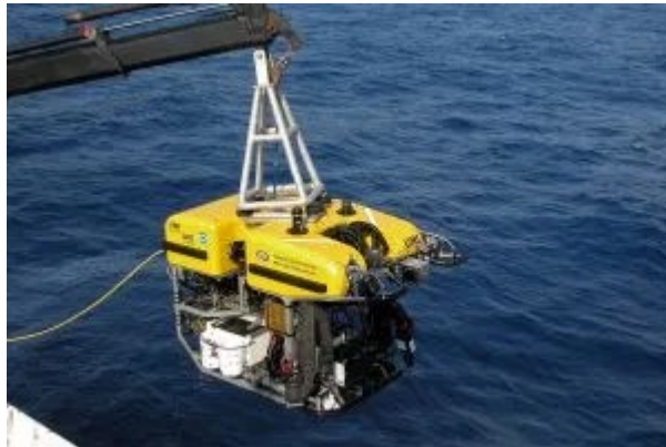
நீர்மூழ்கி எந்திரன்
