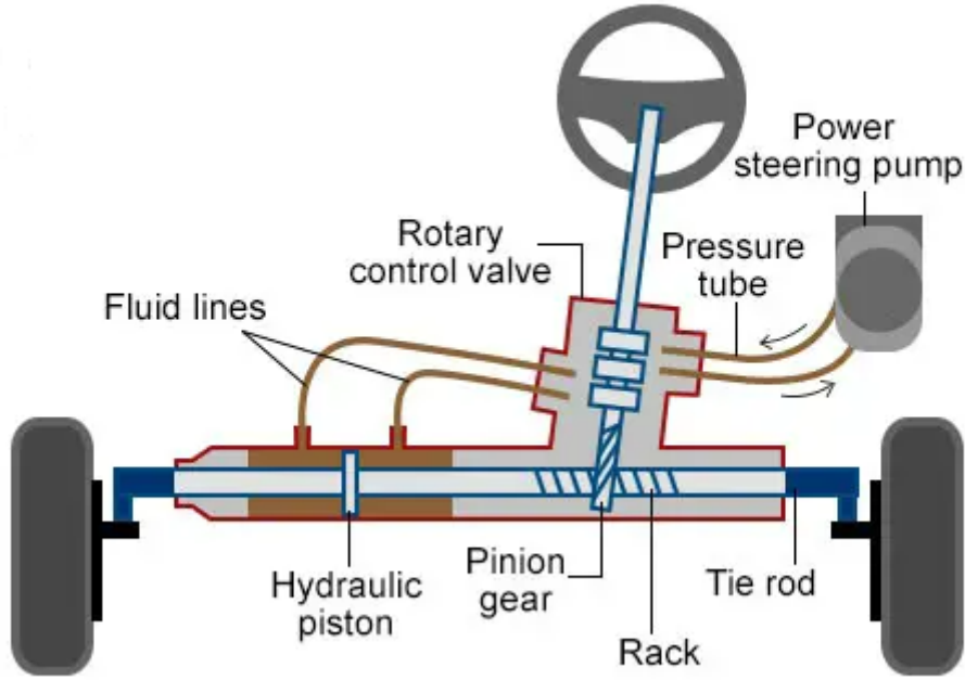
நீரழுத்த திறன் உதவித் திருப்பல்
