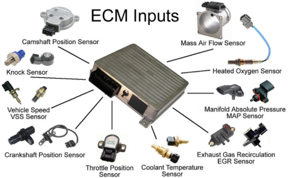
பொறிக் கட்டுப்பாட்டக உணரிகள்
