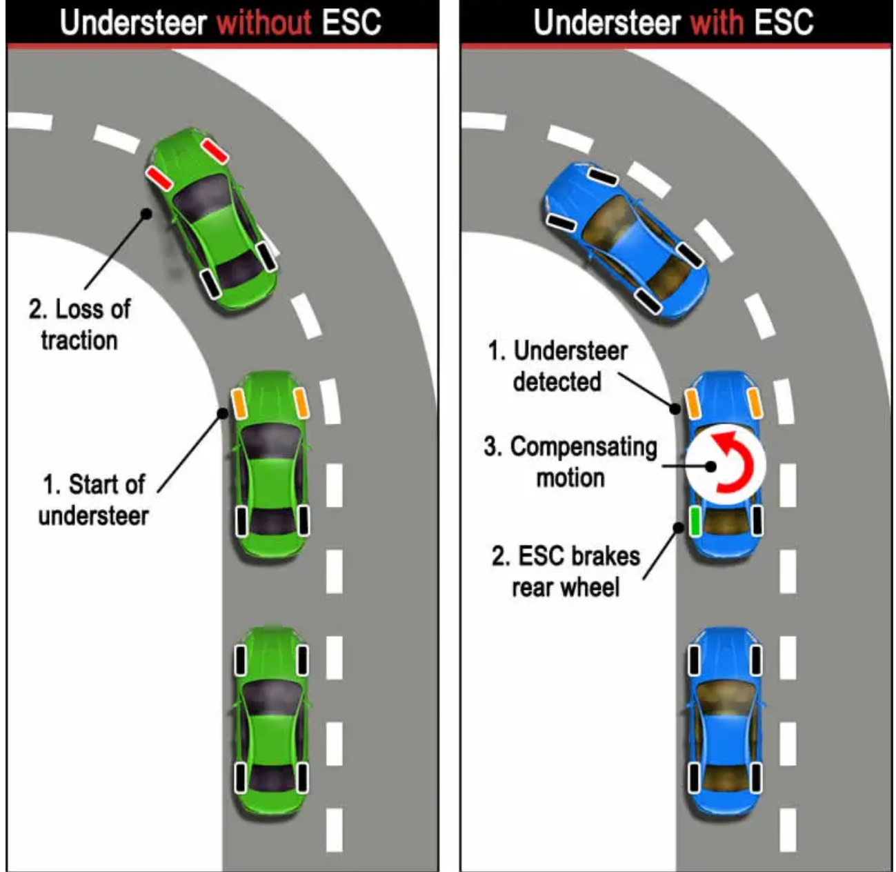
மின்னணு நிலைத்தன்மை கட்டுப்பாடு
