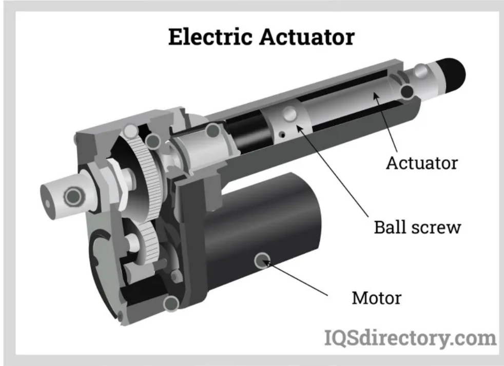
மின் நேரியல் இயக்கி வெட்டுத் தோற்றம்
